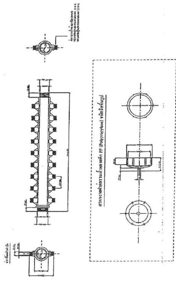
ภาพขยายของรอกพลาสติก PP (Polypropylene) ชนิดถักขึ้นรูป
