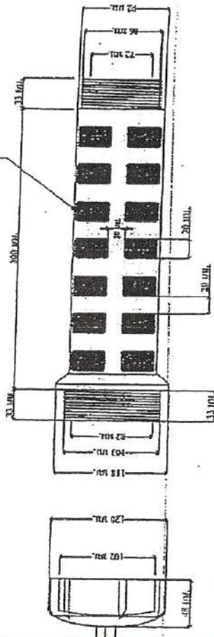
ภาพขยายของกระจ่ายน้ำพลาสติก PP (Polypropylene) ชนิดสี่ชั้นรูป
